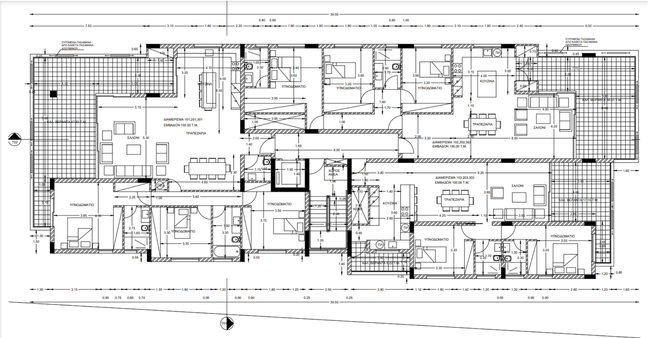
ΚΑΤΟΨΗ ΤΥΠΙΚΟΥ ΟΡΟΦΟΥ
