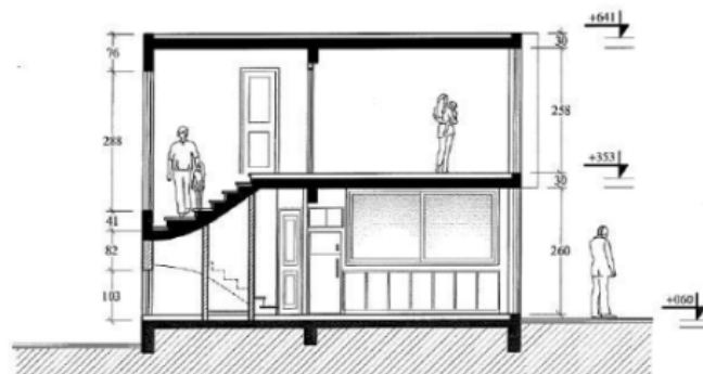
Τομη Α-Α
