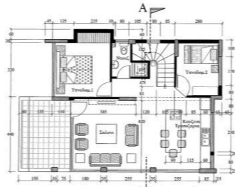
Κατοψη Ισογείου
