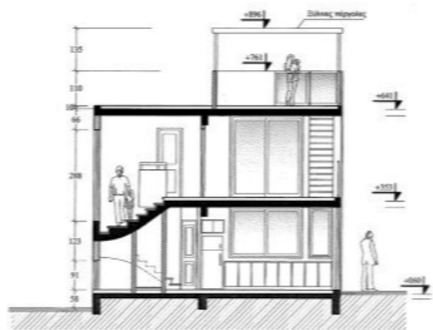
Τομή Α-Α
