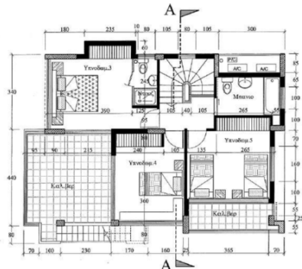
Κατοψη Οροφου
