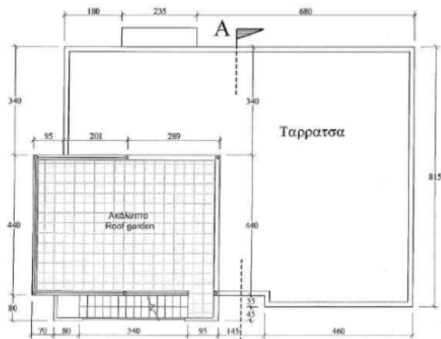
Ανωψη
