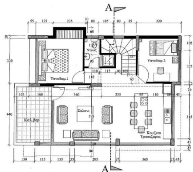
Κατοψη Ισογείου
