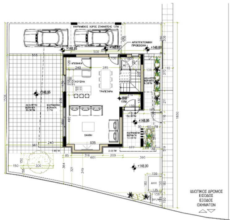
ΚΑΤΟΨΗ ΙΣΟΓΕΙΟΥ
